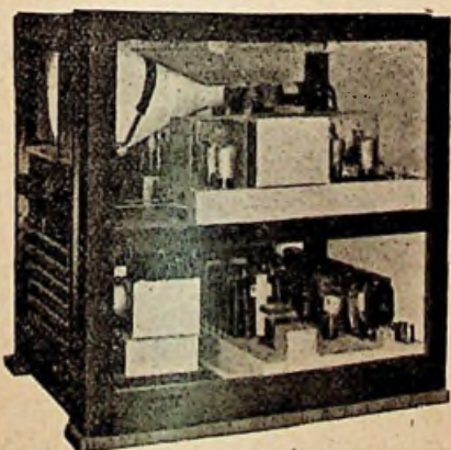
Fig. 2. Het inwendige van het apparaat.
