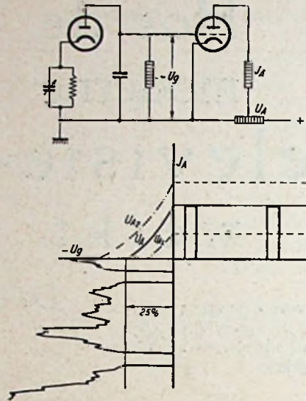
Fig. 5. Schema van de „amplitudezeef” met verklaring van de wijze, waarop de beeldmodulatie buiten het kipapparaat wordt gehouden en alleen de draaggolfonderbrekingen als synchroniseerimpulsen aan het kipapparaat worden doorgegeven.
