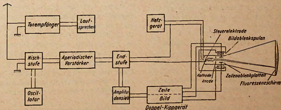
Fig. 3. Blokschema van den Lorenz-televisieontvanger, met kleine wijziging ontleend aan M. von Ardenne's boek Fernsch Empfang.
